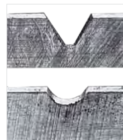
Bild 2: geschliffene Kerben in 2 mm starkem gehärtetem Stahl (60 HRC) oben: mit DEGUSSIT-Feile unten: mit gebundener Feile.
